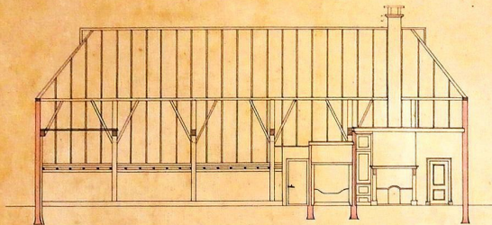
Zijaanzicht.
